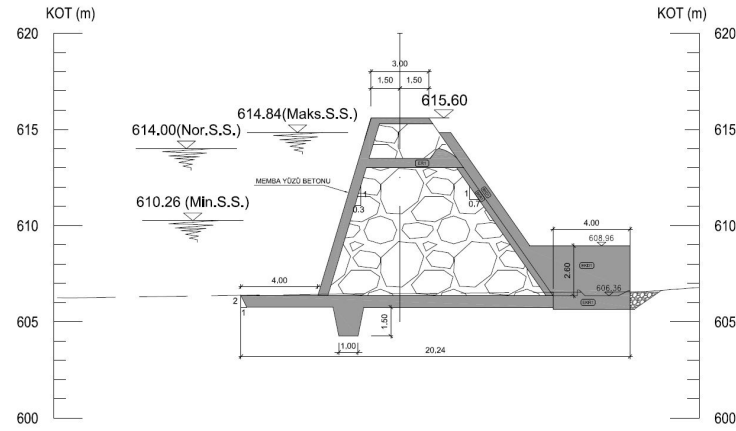
KESİT-B10 (KM:0+100.00)
