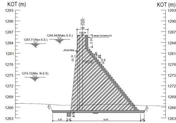
KESİT-B3 (KM 0+060.00)
